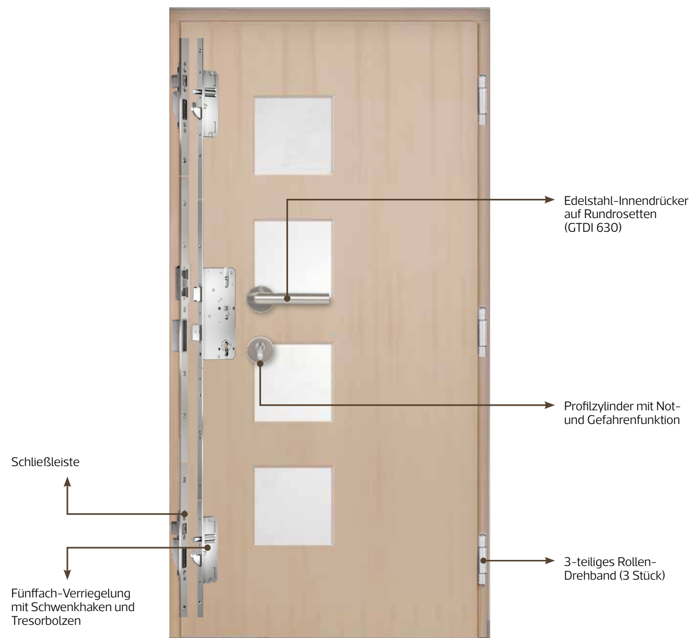
Innenansicht / schematisch
