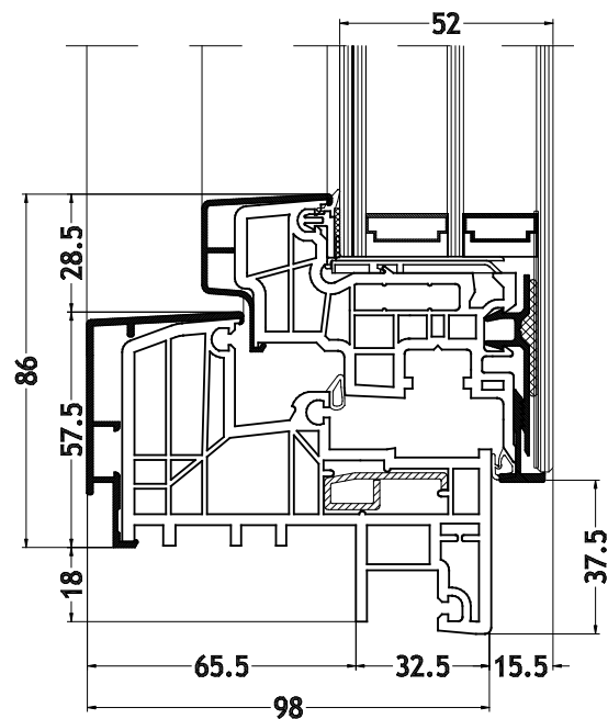
Blendrahmen Z-Form 921N mit Flügel Slim-line Cristal N
