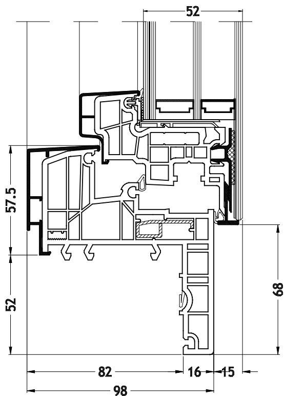
Blendrahmen Z-Form 929N mit Flügel Slim-line Cristal N
