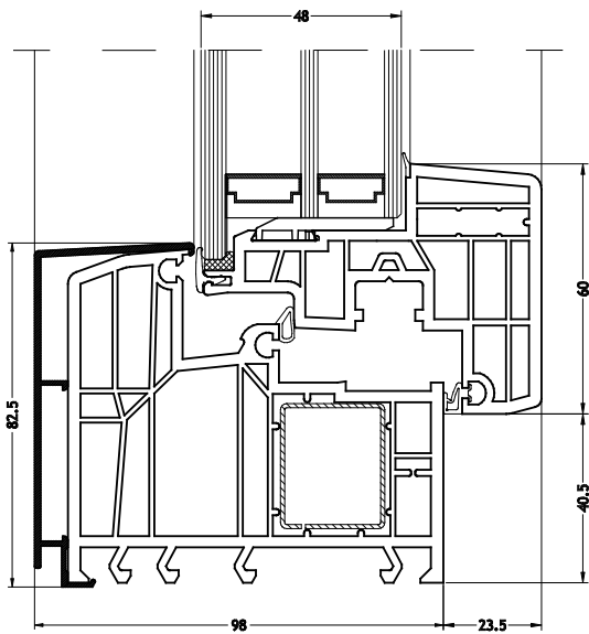
Blendrahmen L-Form 920N mit Flügel Nova-line Plus N
