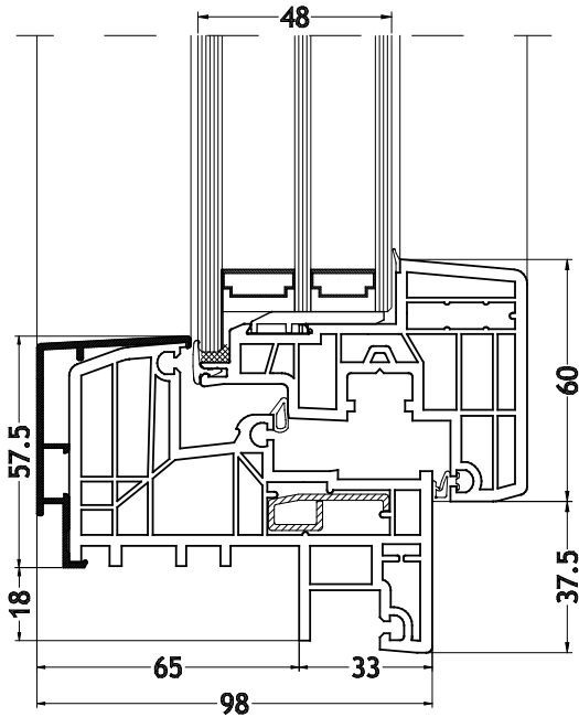
Blendrahmen Z-Form 921N mit Flügel Nova-line Plus N
