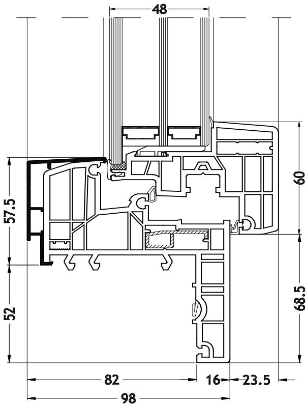
Blendrahmen Z-Form 929N mit Flügel Nova-line Plus N
