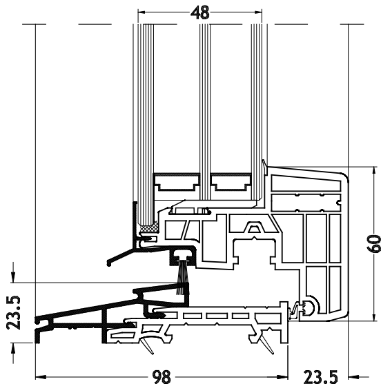
Flache Schwelle mit Flügel Nova-line Plus N
